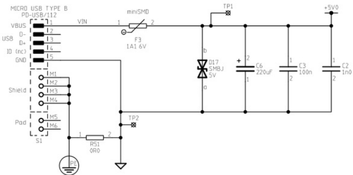
USB Power Input 5V 700mA min
