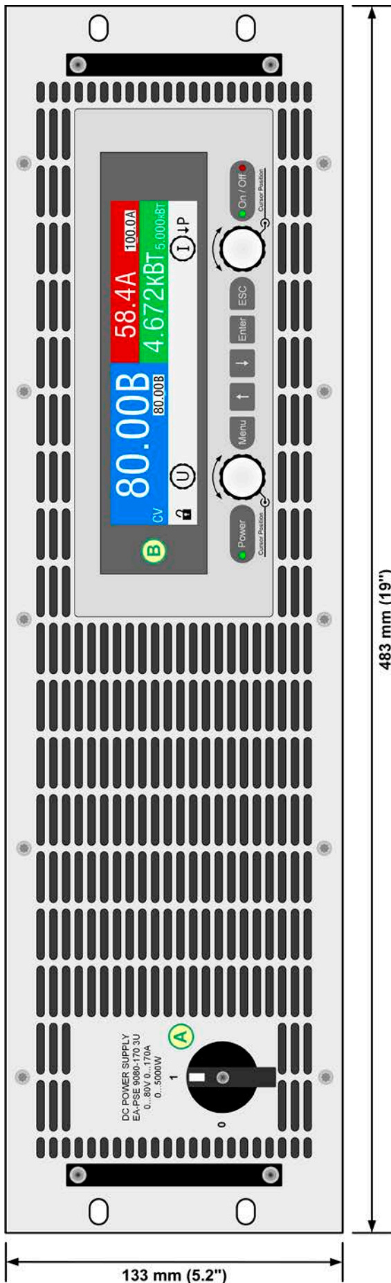
Рисунок 1 - Передняя сторона
